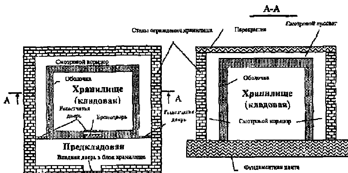
Рисунок П8.1 - Схематичное устройство хранилища ценностей
